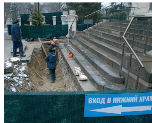
Укрепление фундамента здания собора. 2011 г.
